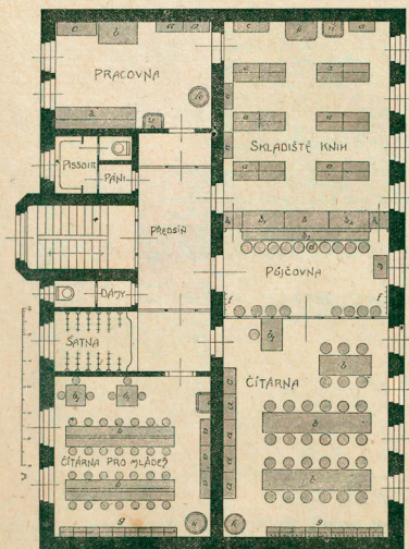
Pádorys a vnitřní úprava knihovny a čítárny. Vzor č. 22.
