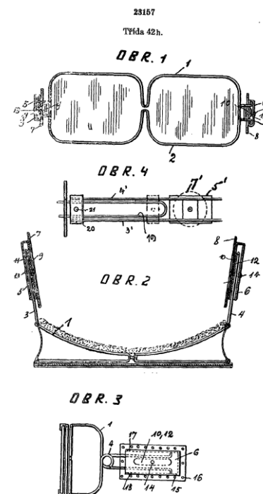
Patent č.23157 Ochranné brýle např. pro automobilisty
